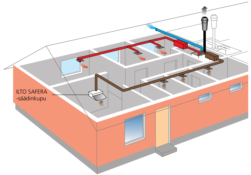
LTO-laitteen ohjaus liesikuvusta asuntokohtaisessa ilmanvaihdossa
